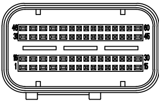
电子控制模块 (ECM) OEM线束接头配合面
