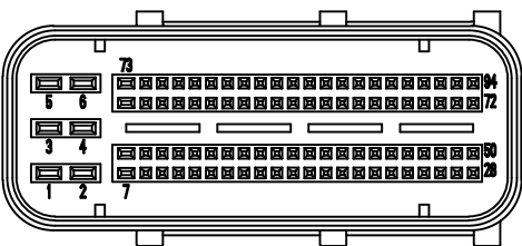
电子控制模块 (ECM) OEM线束接头配合面
