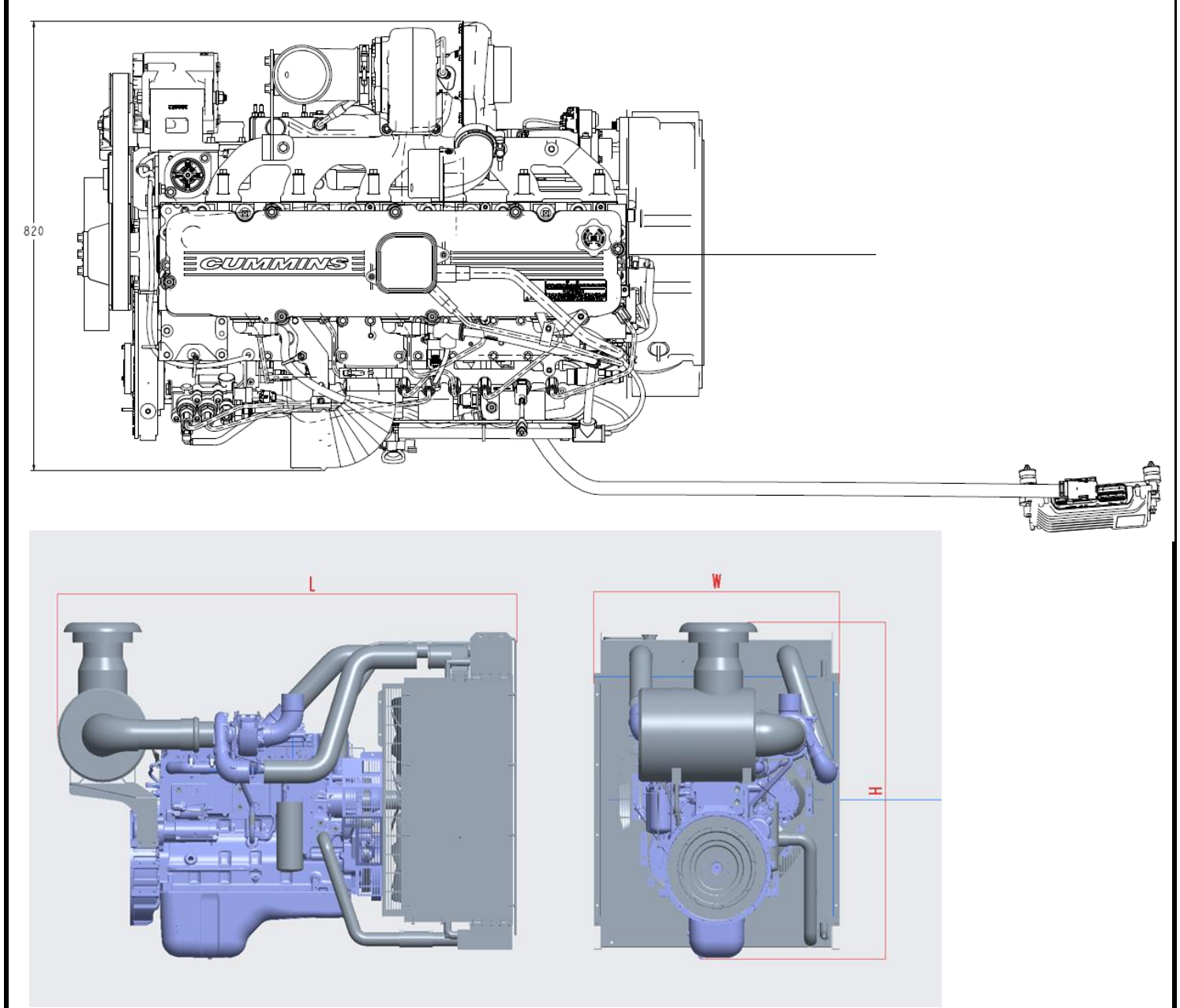
发动机及动力单元尺寸数据
