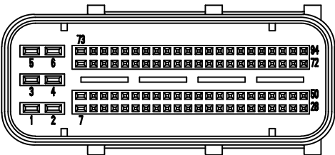
诊断接头 接头配合面
