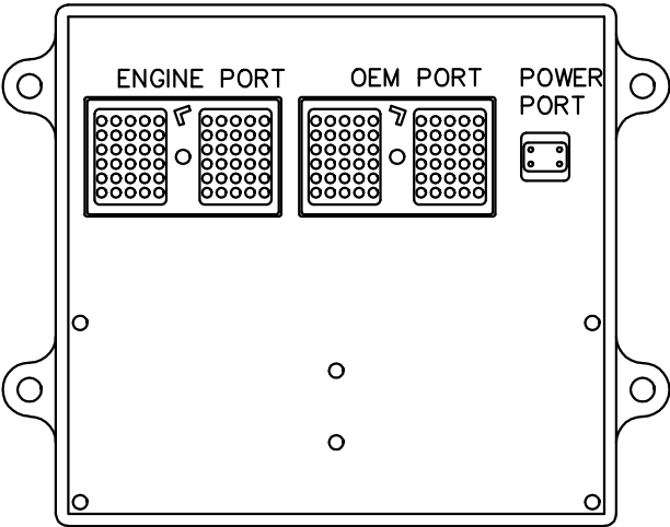
ELECTRONIC CONTROL MODULE (ECM) ECM 电子控制模块
